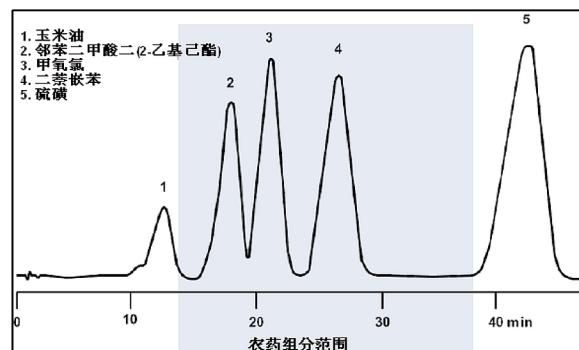
图 1. US EPA 3640A 方法的校正样的环己烷/乙酸乙酯（1:1, v/v）色谱图
